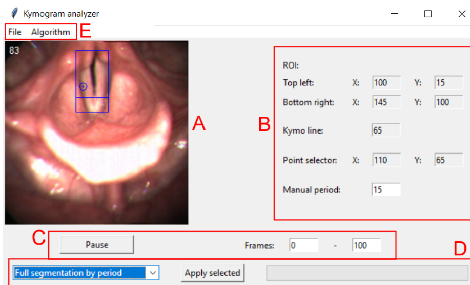
Obrázek 7.1: Hlavní okno aplikace.
