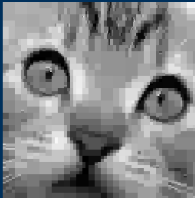
Haarova báze, rekonstrukce z 1/64 celkového množství původních koeficientů (zachovány koeficienty s největší absolutní hodnotou, viz snímek 51)
