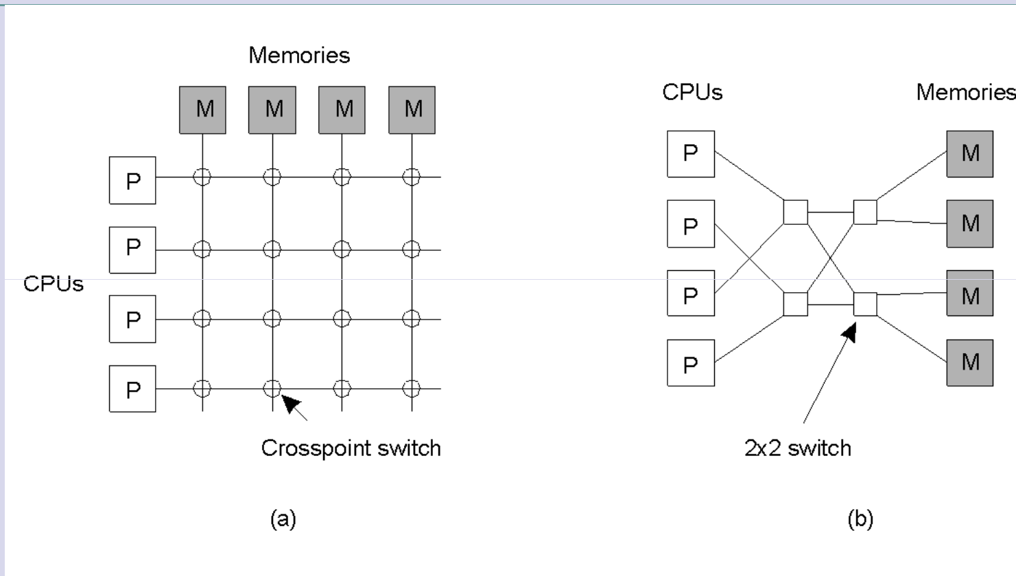
a) Křížový přepínač
